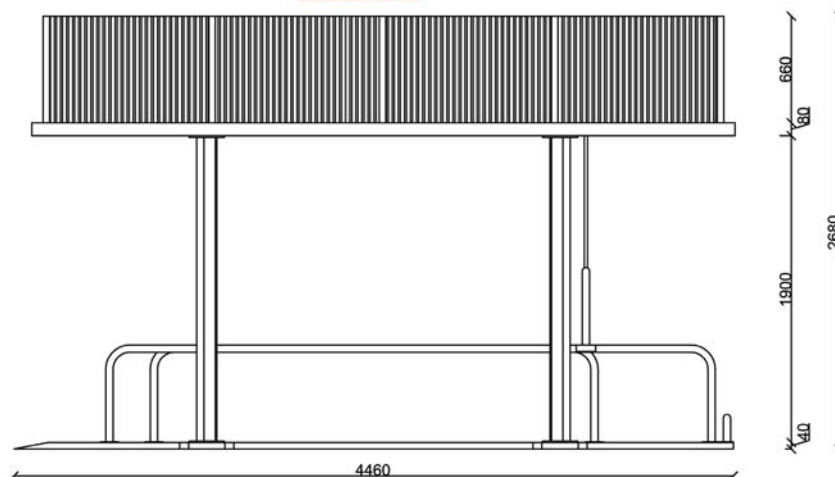
VISTA LATERALE
